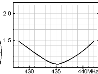
VSWR特性
