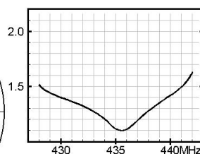
VSWR 特性
