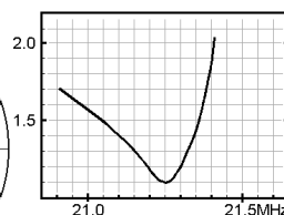
< VSWR 特性 >
