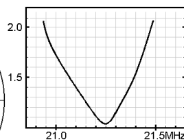
< VSWR 特性 >
