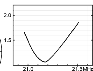
VSWR
