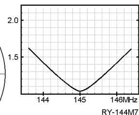
VSWR 特性
