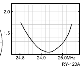
VSWR 特性
