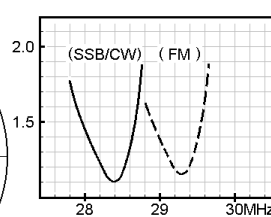
VSWR 特性
